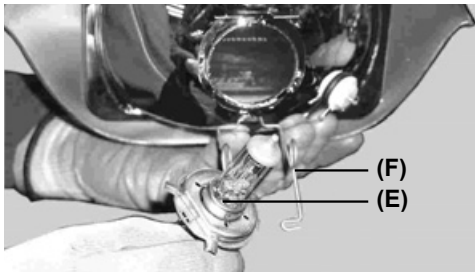
(F). Alambres de sujeción de la bombilla.
